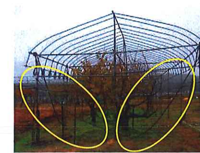
写真 30 沈降力により変形した筋交いパイプ
