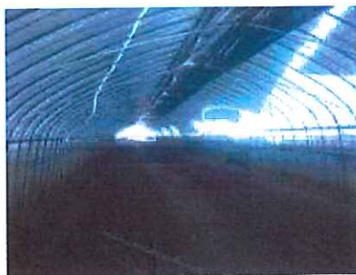
写真 34 無加温ハウスで、ハウス密閉により屋根面の雪が滑落している状況
